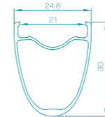
24.6mm幅のタフなワイドリム
