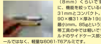
マルチ5は、軽量な6061-T6アルミです。
