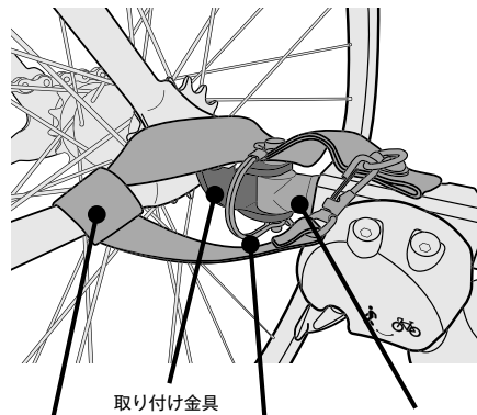
セーフティストラップ 取り付け金具 固定用ピン
